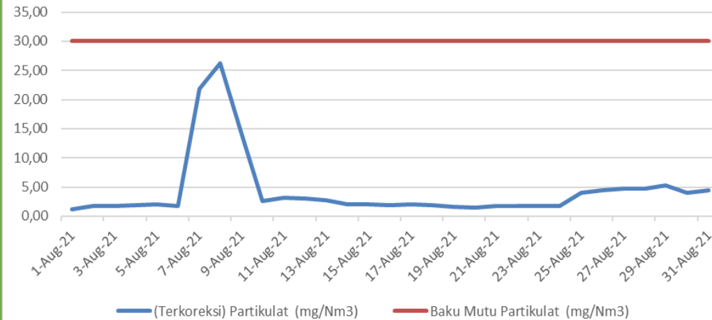
PEMBACAAN HASIL PENGUKURAN CEMS PARTIKULAT HRSG 3.1 PT. INDONESIA POWER BULAN AGUSTUS 2021
