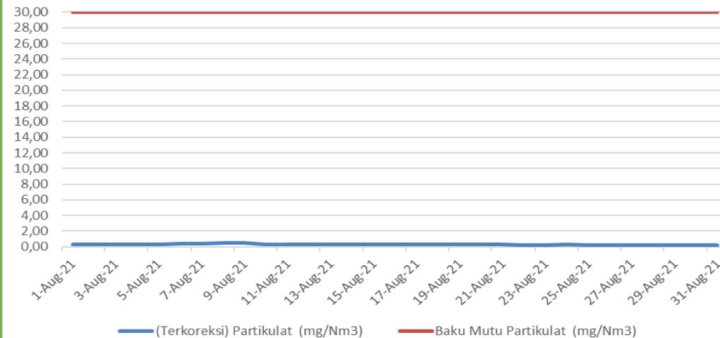
PEMBACAAN HASIL PENGUKURAN CEMS PARTIKULAT HRSG 4.1 PT. INDONESIA POWER BULAN AGUSTUS 2021
