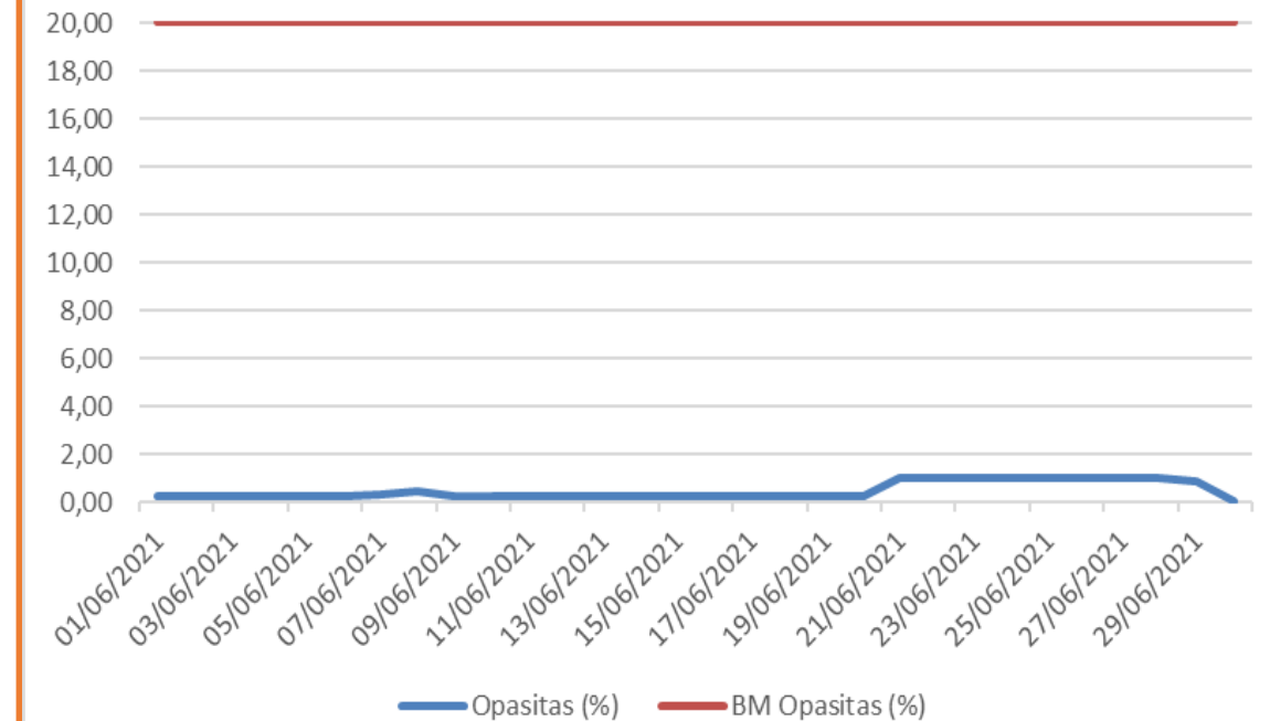
PEMBACAAN PENGUKURAN CEMS OPASITAS PT. JAKARTA CAKRA TUNGGAL STEEL MILL BULAN JUNI 2021
