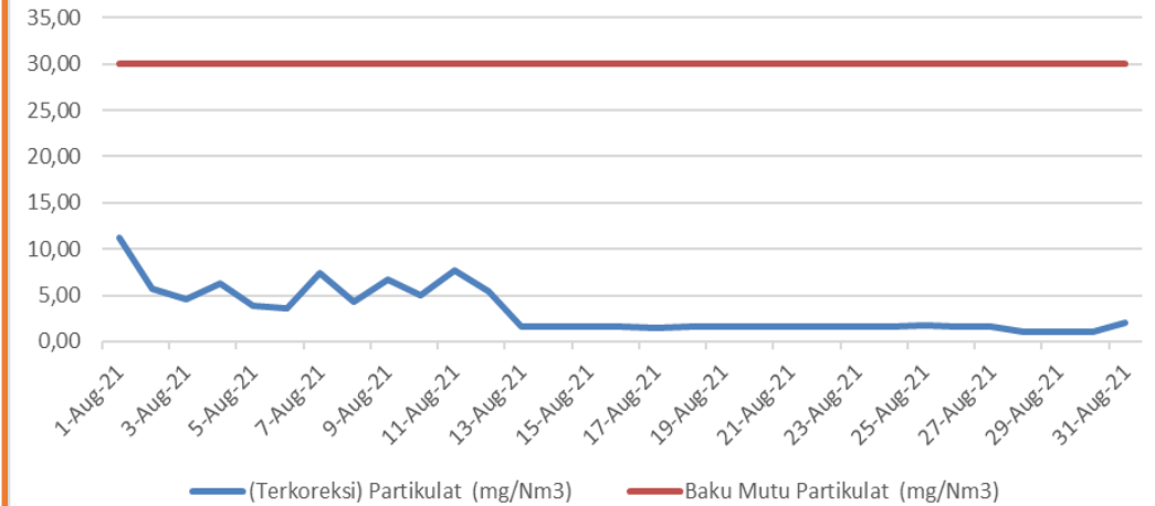
PEMBACAAN HASIL PENGUKURAN CEMS PARTIKULAT HRSG 1.3 PT. INDONESIA POWER BULAN AGUSTUS 2021
