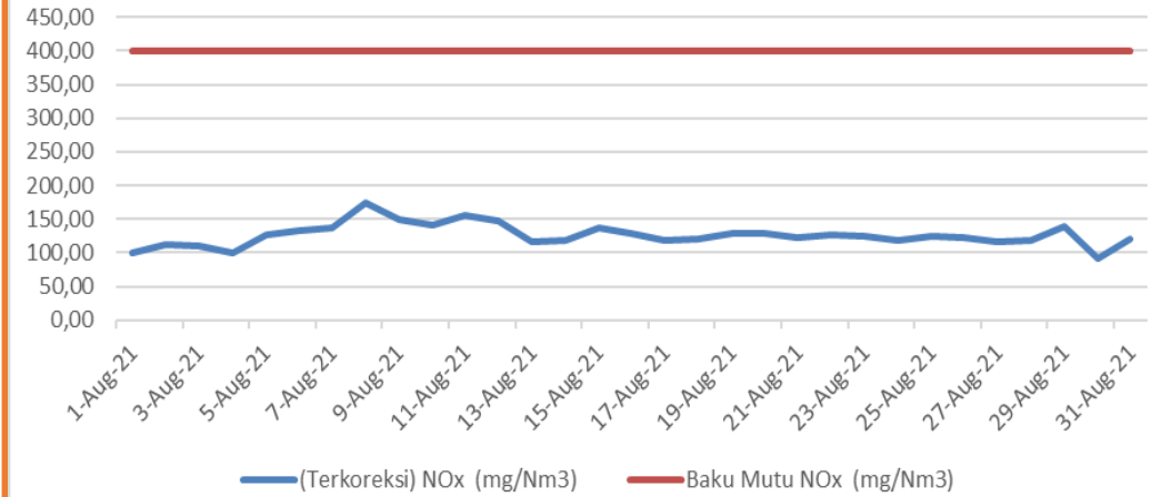
PEMBACAAN HASIL PENGUKURAN CEMS PARAMETER NO x HRSG 3.1 PT. INDONESIA POWER BULAN AGUSTUS 2021
