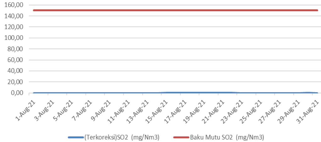
PEMBACAAN HASIL PENGUKURAN CEMS PARAMETER SO 2 HRSG 4.1 PT. INDONESIA POWER BULAN AGUSTUS 2021
