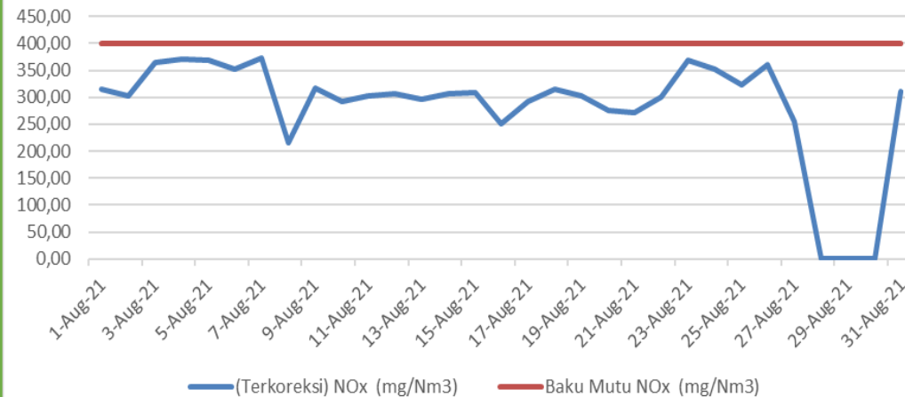
PEMBACAAN HASIL PENGUKURAN CEMS PARAMETER NO x HRSG 1.3 PT. INDONESIA POWER BULAN AGUSTUS 2021
