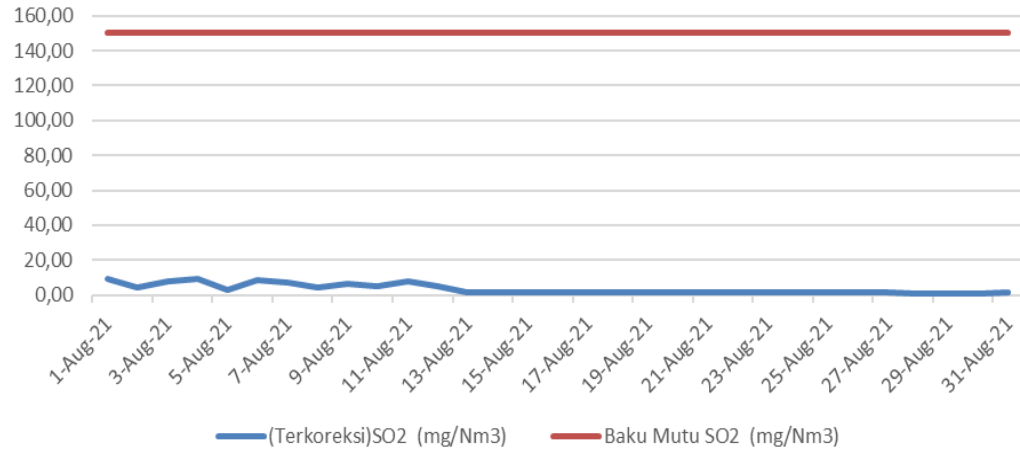
PEMBACAAN HASIL PENGUKURAN CEMS PARAMETER SO 2 HRSG 1.3 PT. INDONESIA POWER BULAN AGUSTUS 2021
