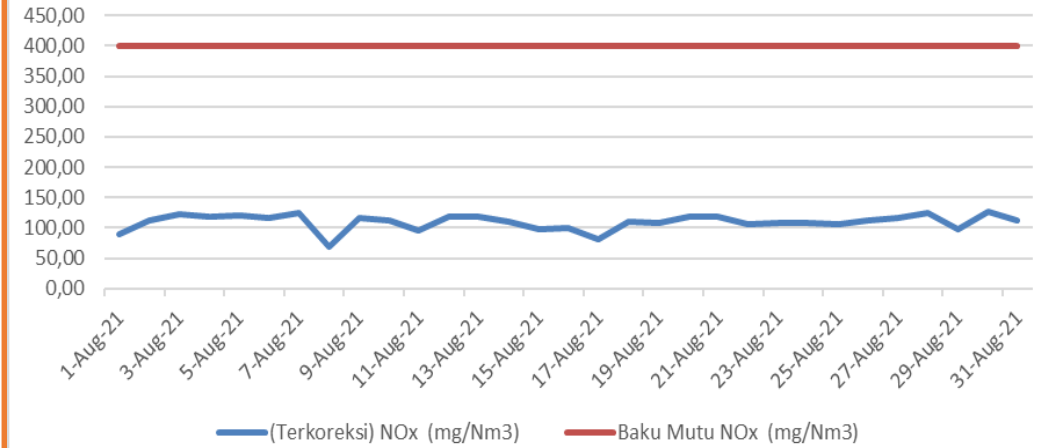
PEMBACAAN HASIL PENGUKURAN CEMS PARAMETER NO x HRSG 4.1 PT. INDONESIA POWER BULAN AGUSTUS 2021
