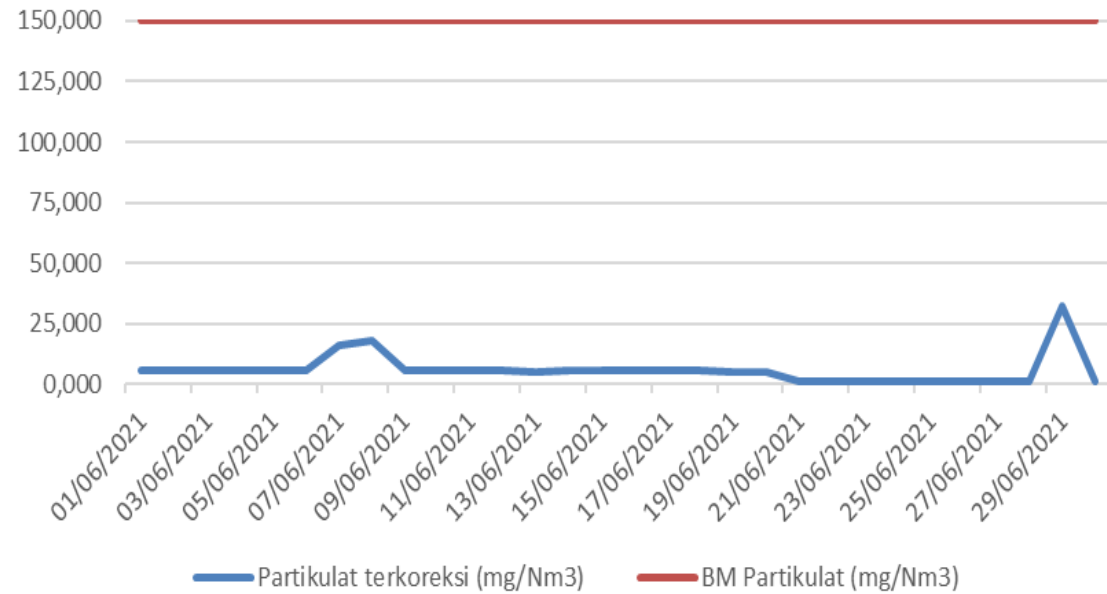
PEMBACAAN HASIL PENGUKURAN CEMS PARAMETER PARTIKULAT PT. JAKARTA CAKRA TUNGGAL STEEL MILL BULAN JUNI 2021
