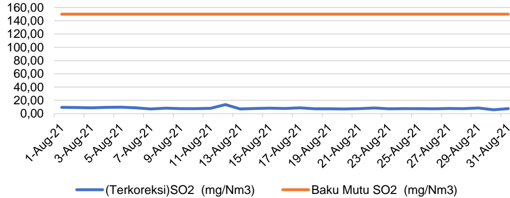
PEMBACAAN HASIL PENGUKURAN CEMS PARAMETER SO 2 HRSG 3.1 PT. INDONESIA POWER BULAN AGUSTUS 2021
